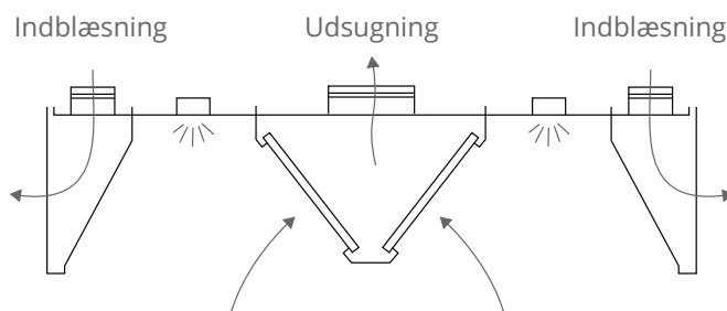
V-format, plantegning
