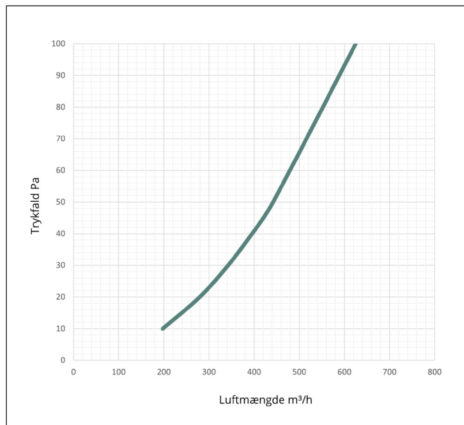
Kapacitetskurve 14 % perforering, K-faktor 62,5 500 mm indblæsning, højde 500 mm
