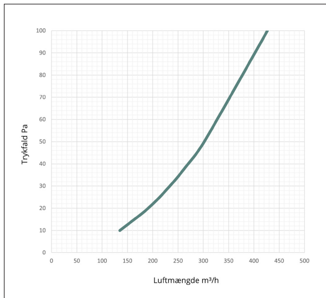
Kapacitetskurve 10 % perforering, K-faktor 42,7 500 mm indblæsning, højde 500 mm
