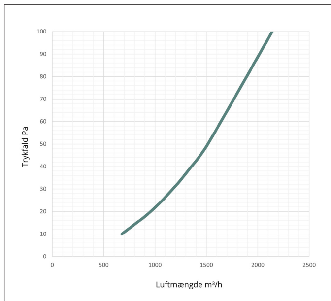
Kapacitetskurve 25 % perforering, K-faktor 214 500 mm indblæsning, højde 500 mm
