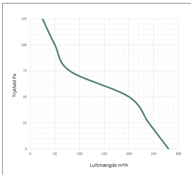
Kapacitetskurve Model A, Ø 125 mm
