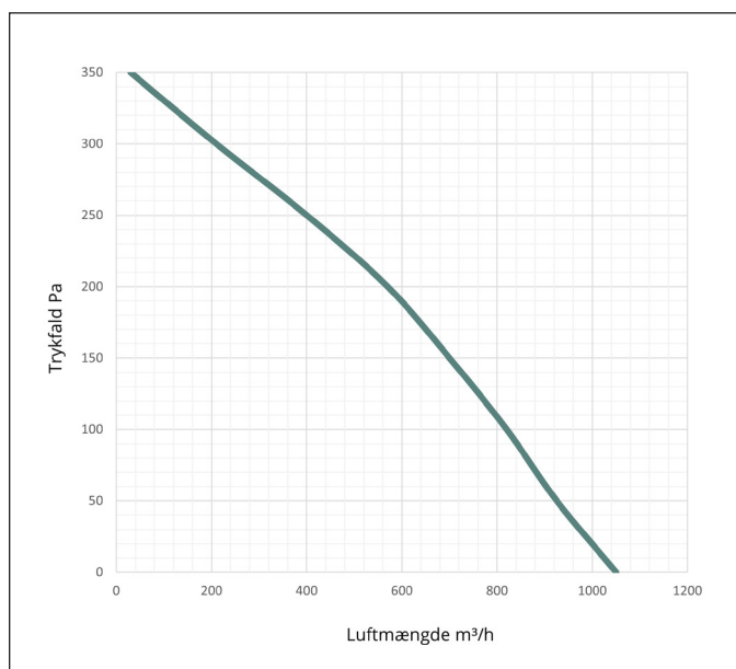
Kapacitetskurve Model C, Ø 200 mm
