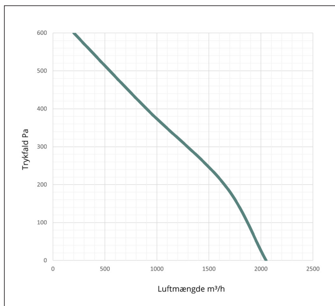
Kapacitetskurve Model E, Ø 315 mm
