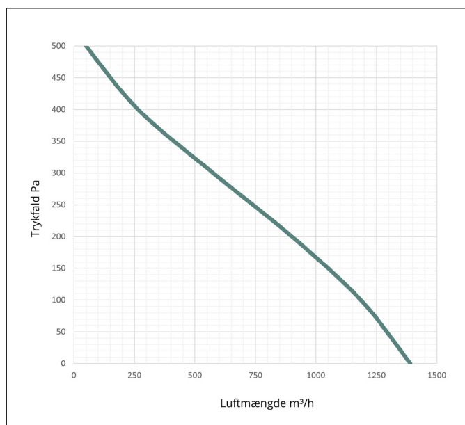
Kapacitetskurve Model D, Ø 250 mm
