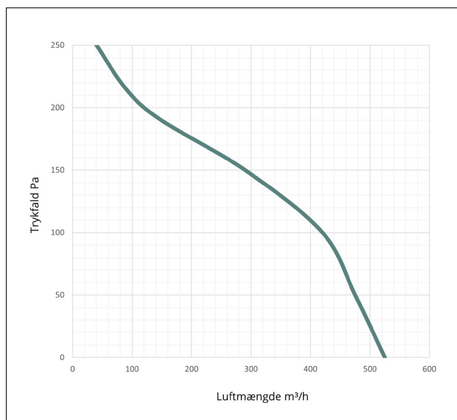
Kapacitetskurve Model B, Ø 160 mm
