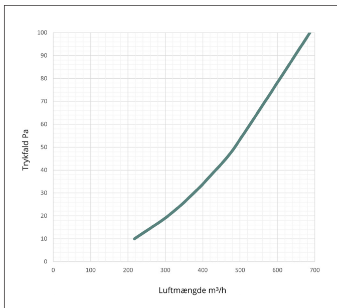
Kapacitetskurve Model A, K-faktor 68,7
