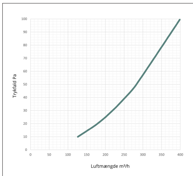
Kapacitetskurve Model A, K-faktor 40
