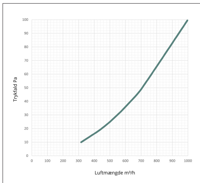
Kapacitetskurve Model B, K-faktor 100
