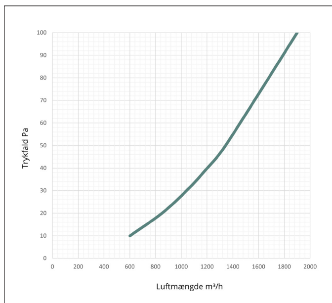
Kapacitetskurve Model C, K-faktor 190
